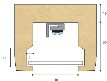
misure in mm mesures en mm
