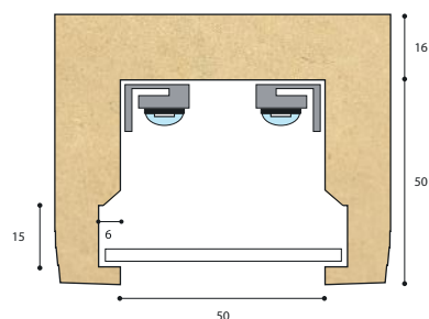
misure in mm mesures en mm
